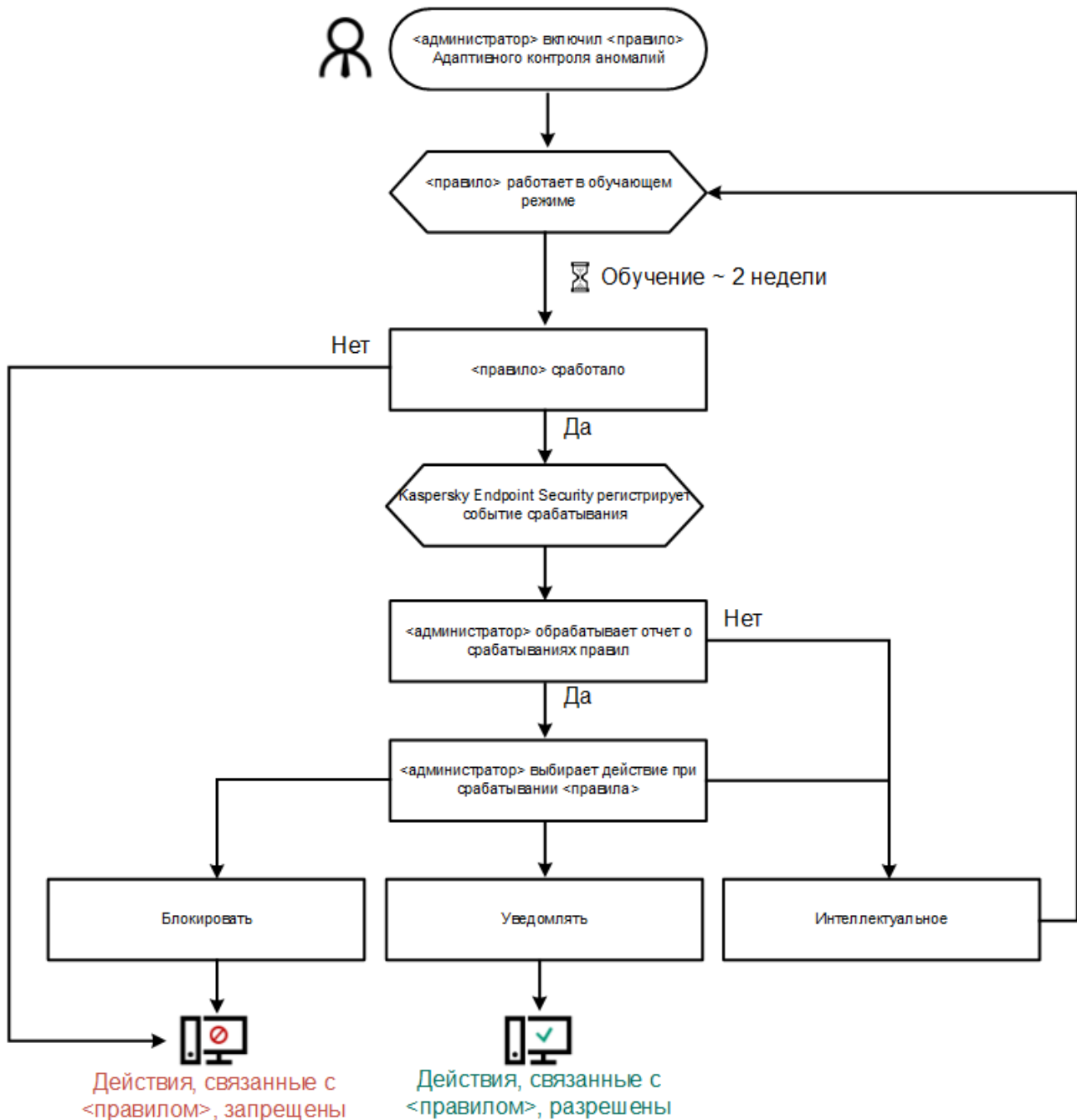
Рисунок 17. Алгоритм работы Адаптивного контроля аномалий
